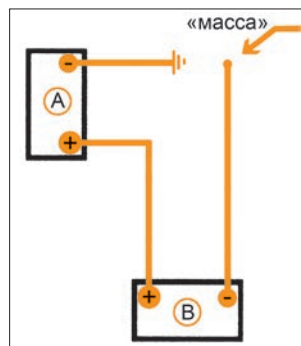
Рис. 21. Схема подключения вспомогательной батареи
